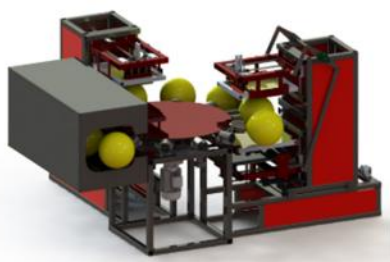
КАР 11 02 Карусельный полуавтомат
