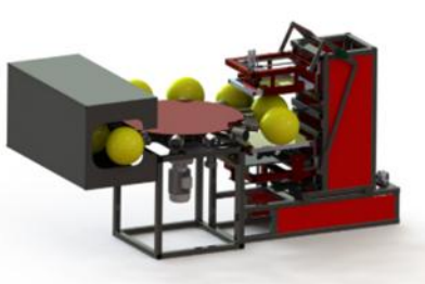
КАР 11 01 Карусельный полуавтомат
